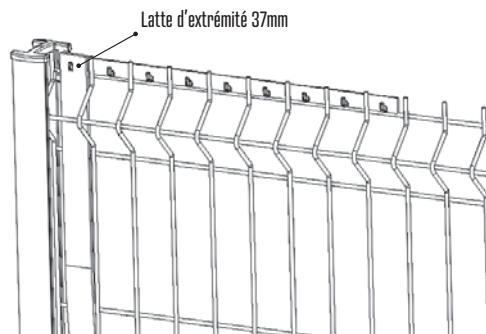
Latte d'extrémité 37mm
